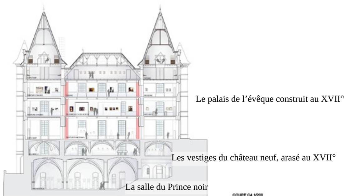
Plan de coupe du musée Ingres Bourdelle, centre de documentation du musée Ingres Bourdelle
