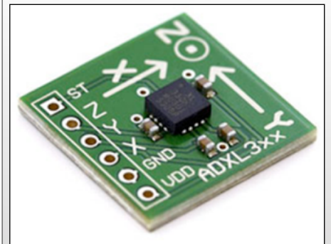
Accéléromètre
